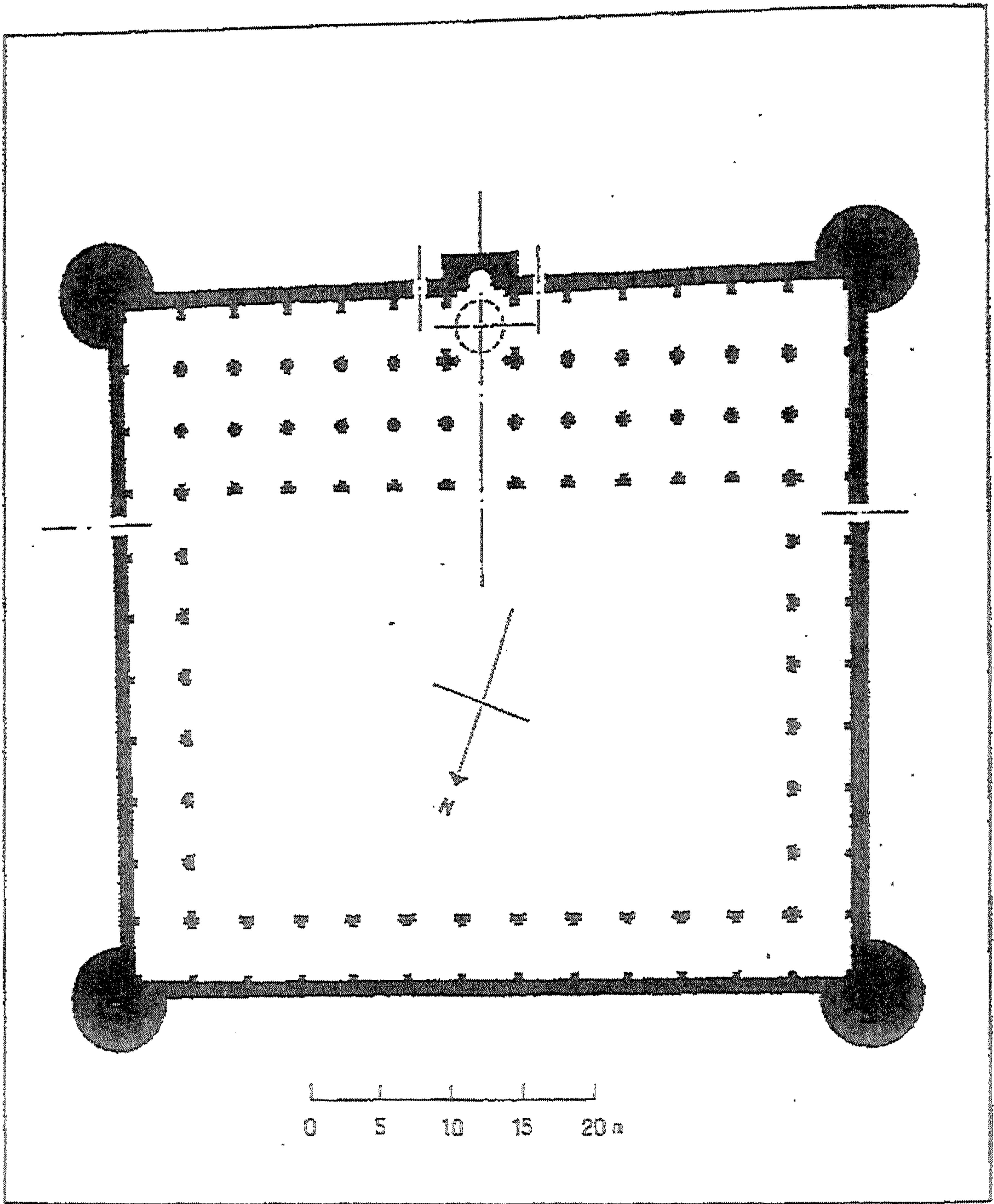
(شكل رقم ٥١) رسم تخطيطي لجامع سوسة بالأبراج الأربعة في عهد الأغلبية عن ليزين.
